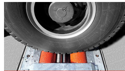
Verstärkter Rollensatz
